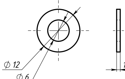
Поз.4 (Шайба паронит)
