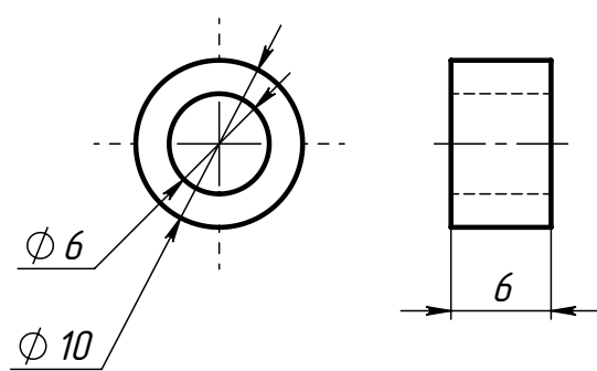
Поз.3 (Втулка паронит)
