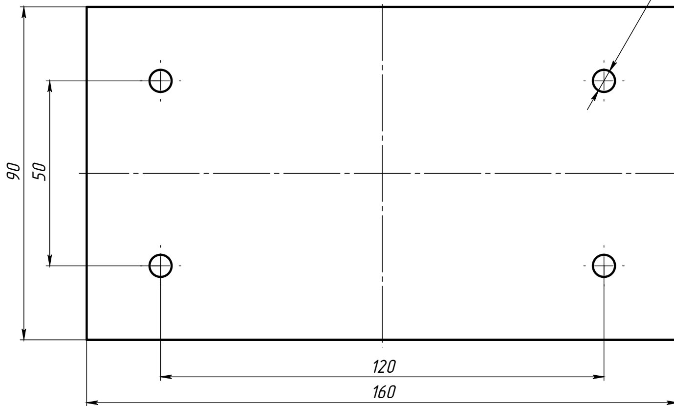
Поз.3 (Втулка паронит)
